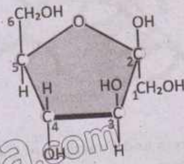
Fructose
