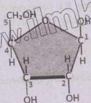
Ribose
