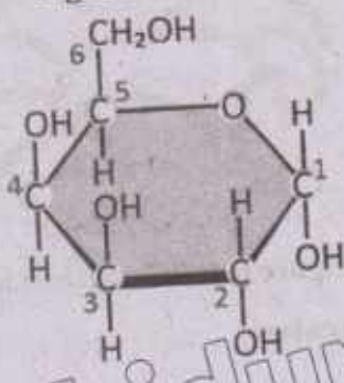
Galactose
