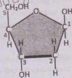
Deoxyribose
