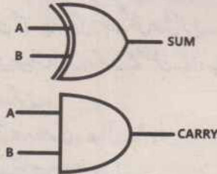
تصویر 3.8: ہاف ایڈر سرکٹ
