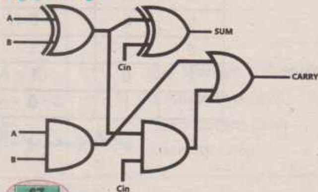
نچل 3.9: فل ایڈر سرکٹ
