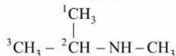
N-methylpropan-2-amine
