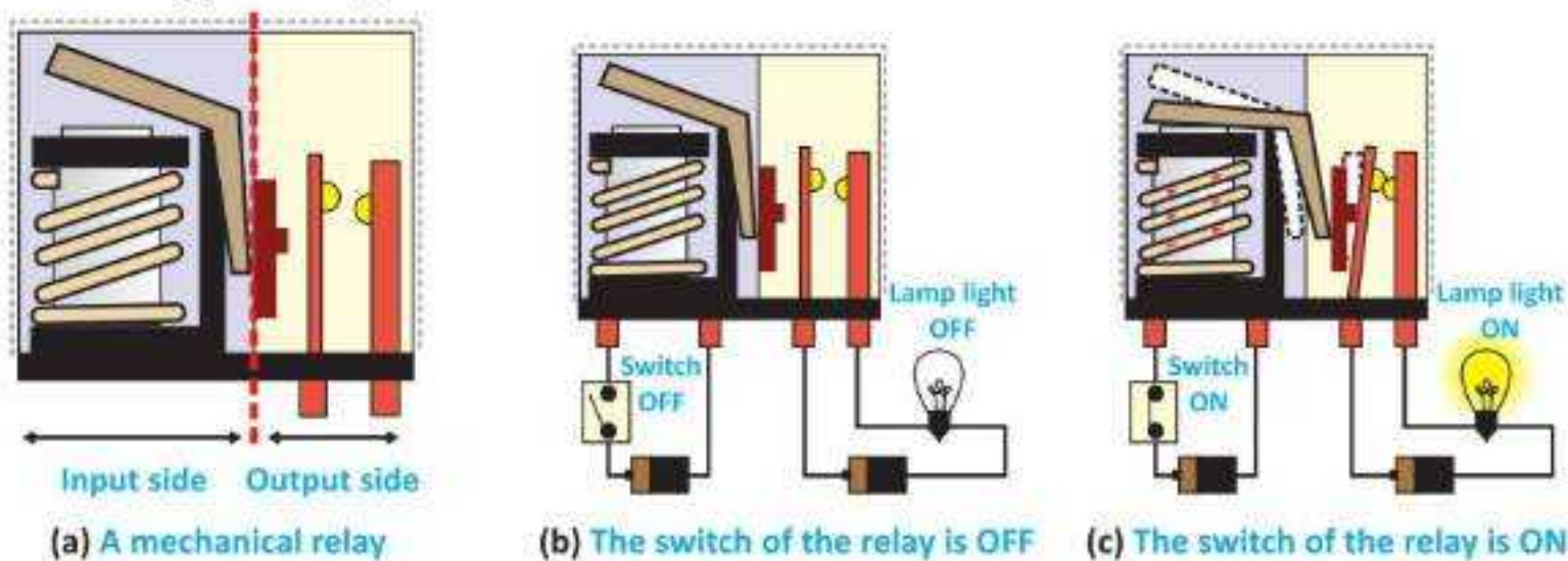
Fig. 17.10: Relay
