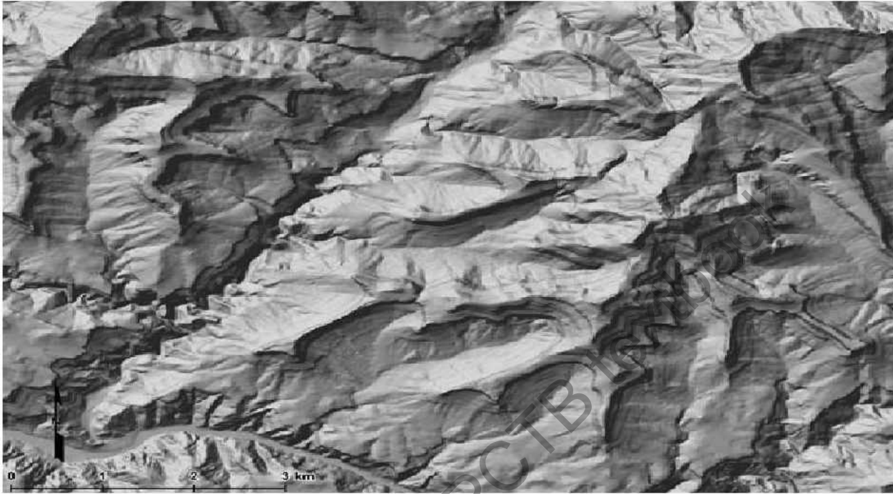
کوہ سائیکس
