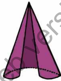
مخروط
