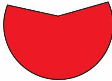
ہموار سطح
