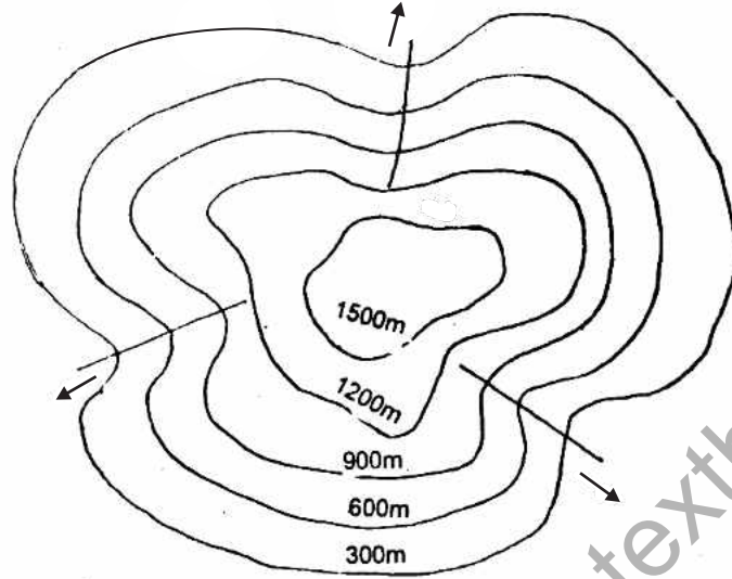
فاصل آب
