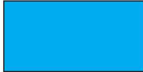
ہموار سطح
