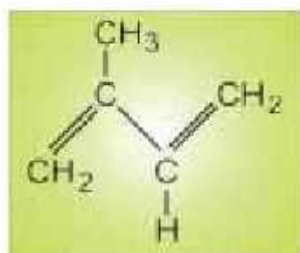
Isoprene unit
