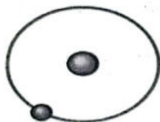
Protium ( {}^1_1\text{H} )
