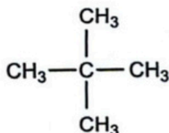
neo-Pentane
