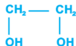
1,2-Ethanediol (Glycol)
