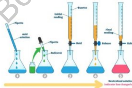
تصویر 7.12 ٹائٹریشن
