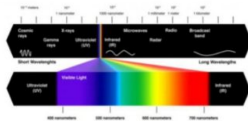
تصویر 7.15 سپیکٹرم
